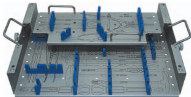
26. Statyw na instrumentarium podstawowe CHARSPINE [40.5299.100] Stand for CHARSPINE basic instrument set Подставка для стандартного набора инструментов CHARSPINE
